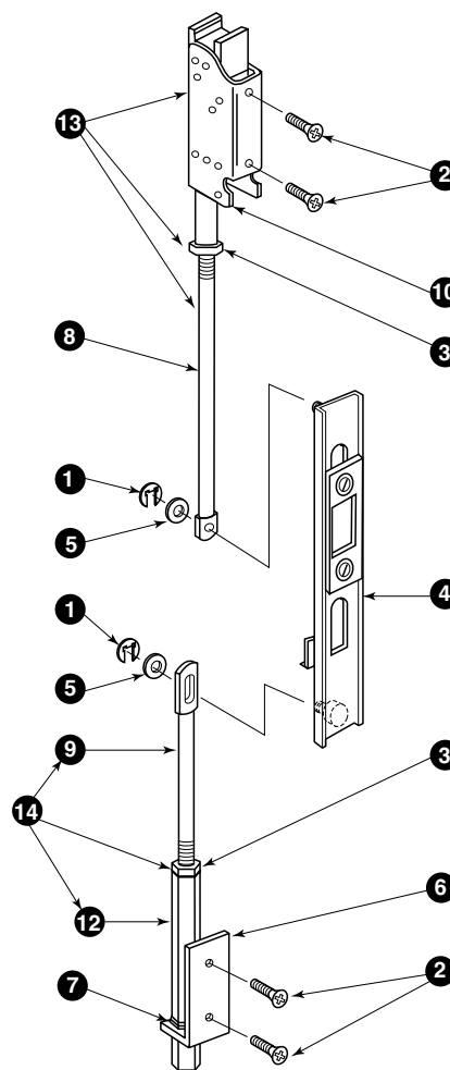
EL rod assembly
